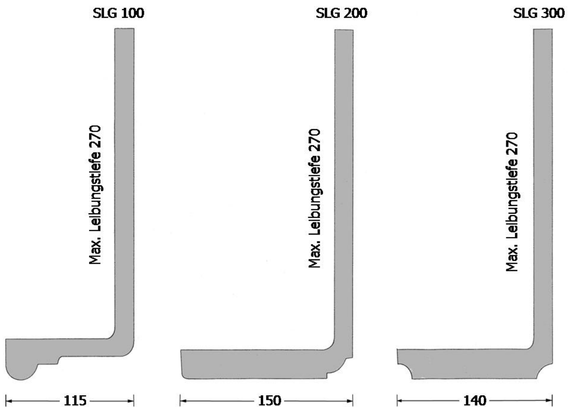
Schalen-Winkelgewände
