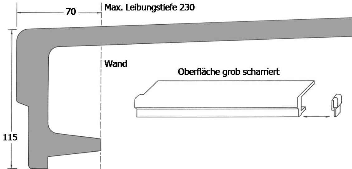
Schalen-Fensterbank SLB 300
