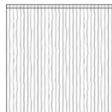
SOP grob-scharriert Oberfläche Platte und Vorderkante grob-scharriert obere waagerechte Kante glatt
