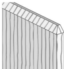
SOP Sockelplatten mit abgeschrägter Vorderkante Dicke Kante oben = 1 cm
