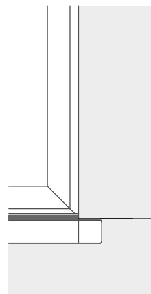
Schalen-Winkelgewände SLG 150 umlaufend mit Schalen-Fensterbank SLB 591
